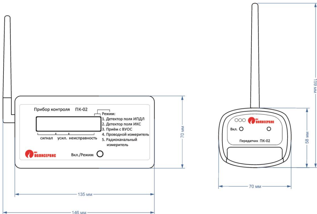
Рисунок 1.1 – Общий вид изделия
