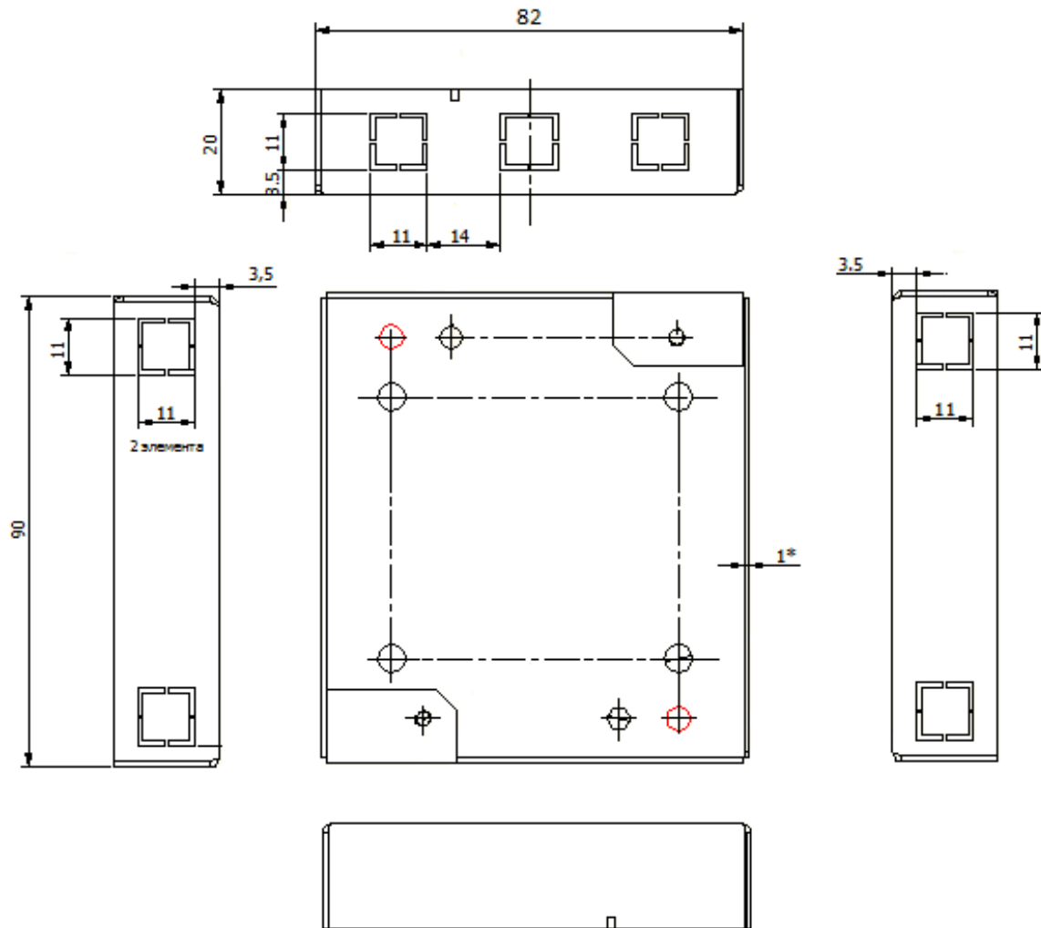
Рисунок 2 - Габаритные размеры коммутационной коробки КК-2757
