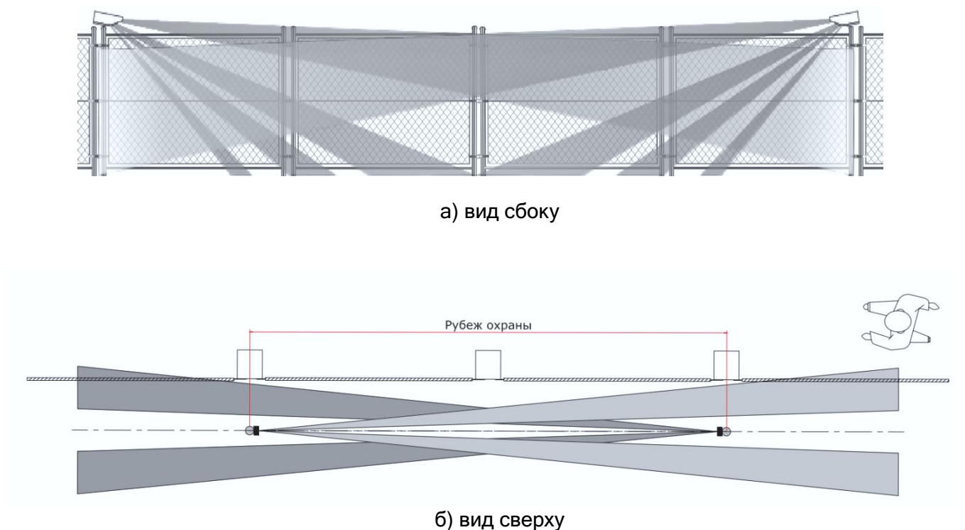
Рисунок 2.2 - Двухнаправленная схема установки извещателей
